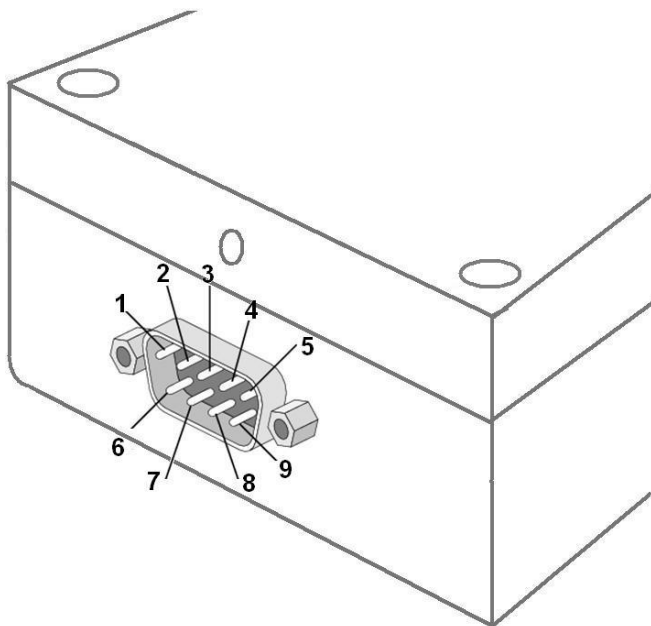
Рис 2. Выводы интерфейсного разъёма
