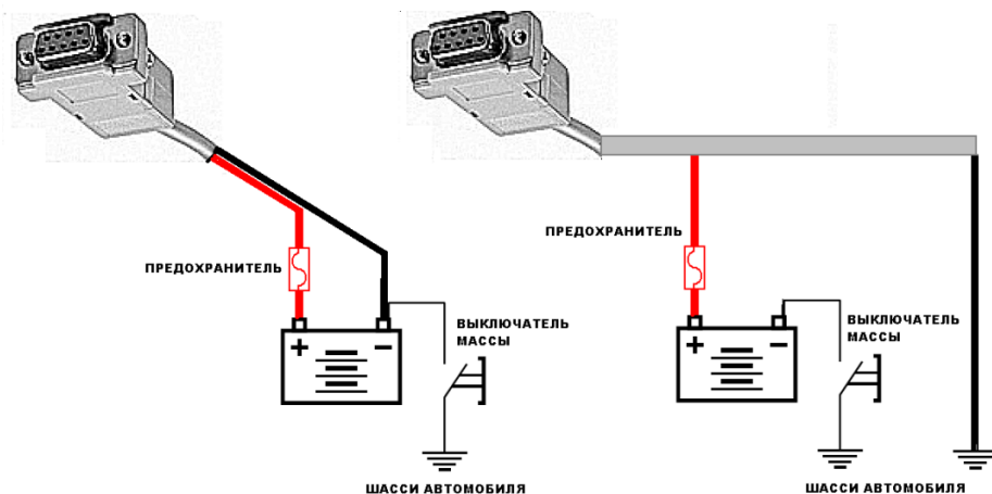
Рис 4. Подключение питания
